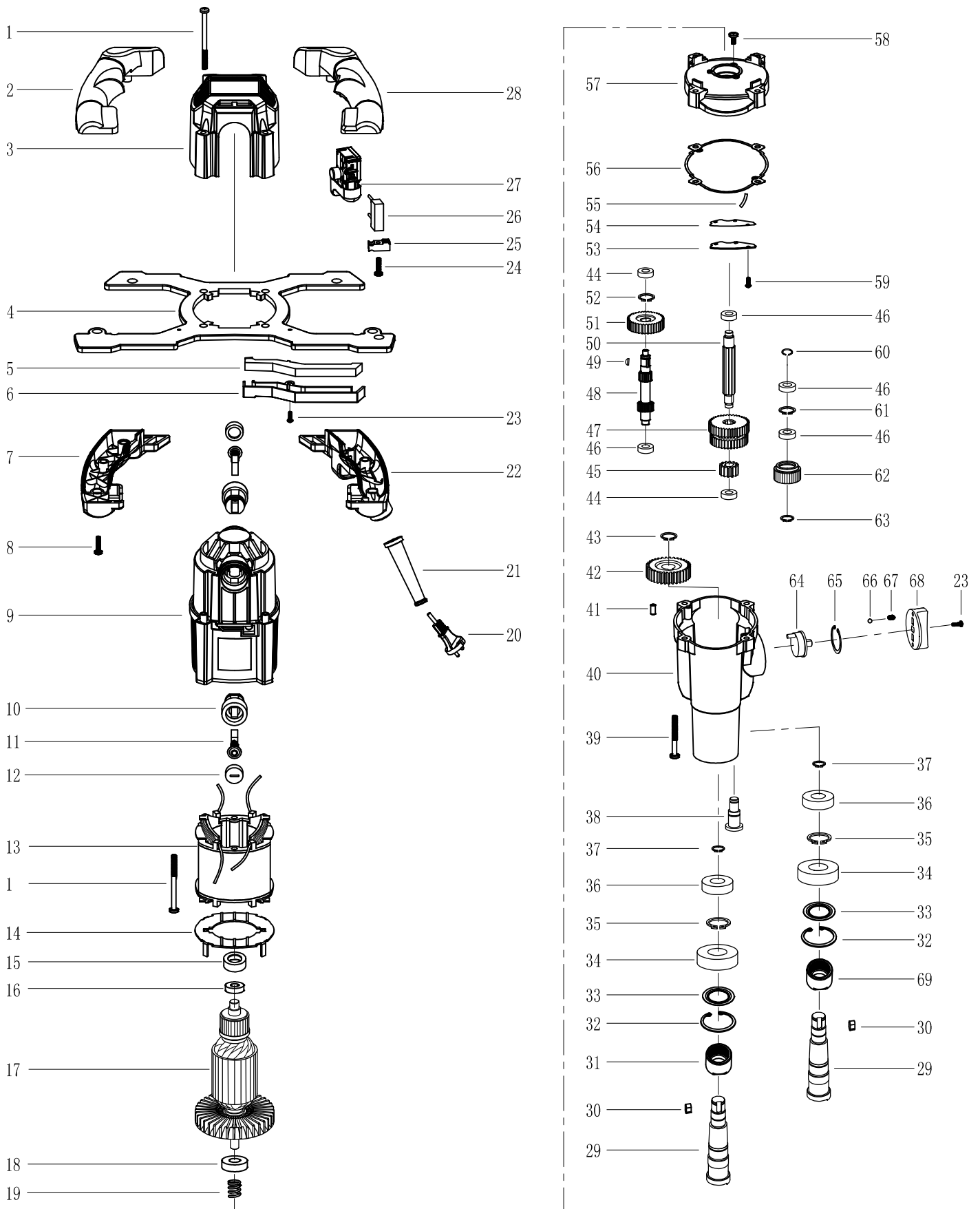
51.03-MD-1800-PRO MÍCHADLO DVOUMETLOVÉ PROFI 1800 W
